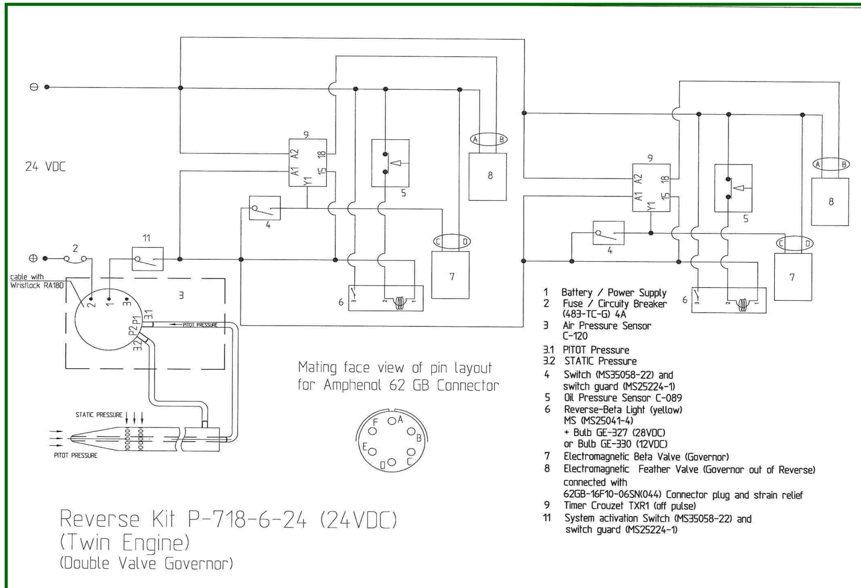
Figure 9 Zweimotorige Flugzeuge: Doppelmagnetventil-Regler - 24 VDC
